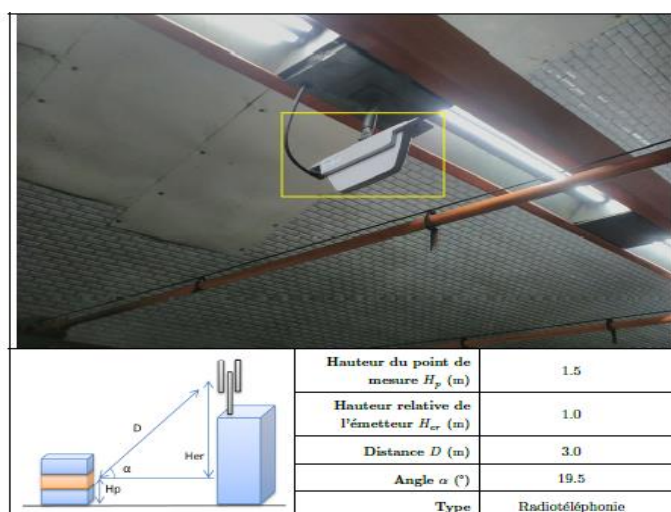
Figure 4. Mesure du point le plus exposé à proximité de l'antenne à la station "Mairie d'Ivry" (Rapport de mesure R_SO9075_1_21)
