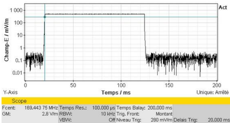
Figure 9 : analyse temporelle du signal émis par le compteur
